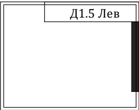
Д1.5Лев Габ.р-р 1390х1090х1000 Сп.место 950х1520
