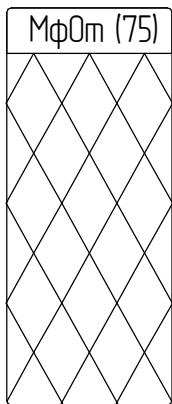
MфОт (75) Габ.р-р 750x1750x970 Сп.место 750x1730
