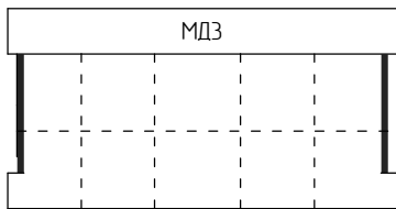
MD3 Габ.р-р 2000x1040x1040 Сп. место: 1920x1480
